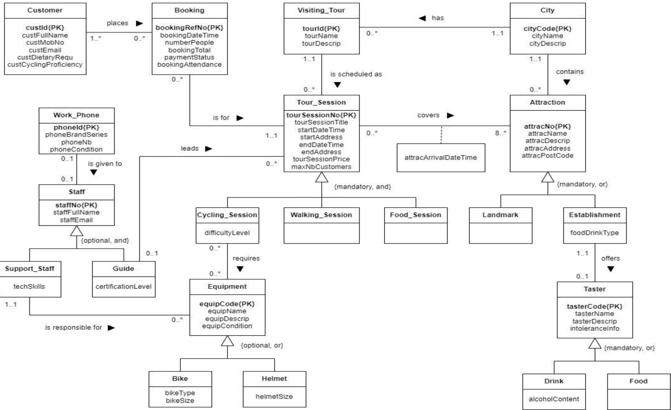
Figure 1. Conceptual EERD for Tourmato
